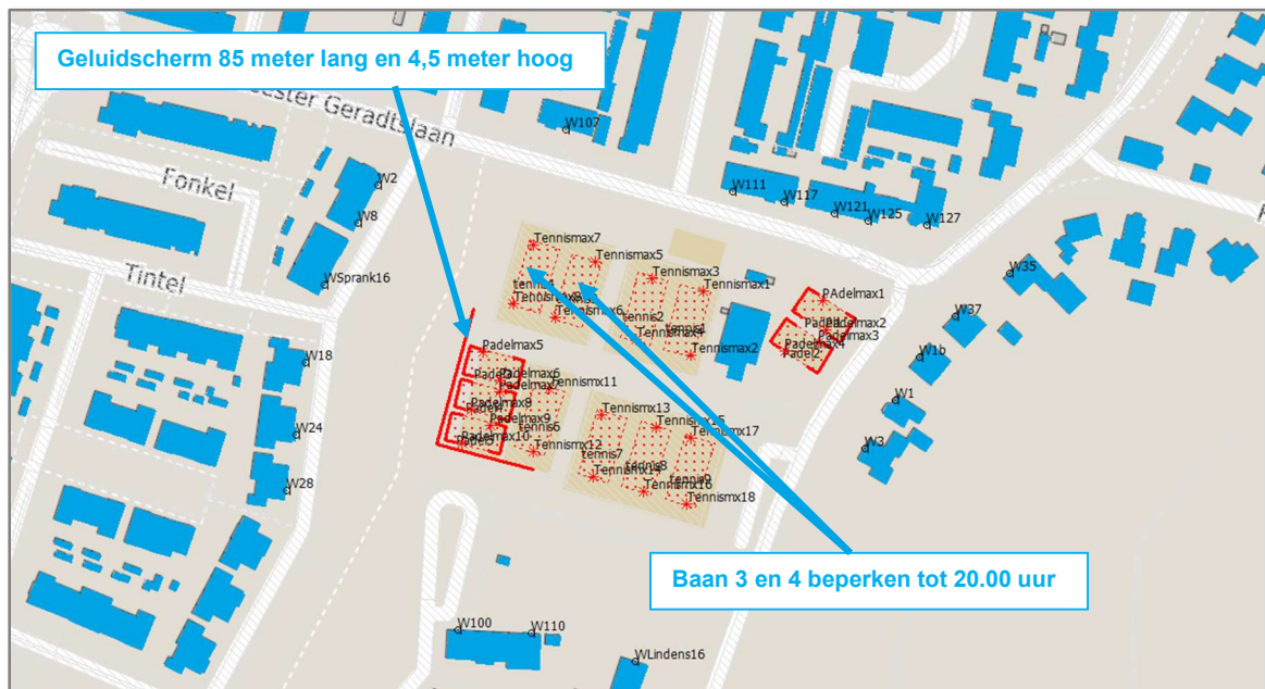
Figuur 3.2 Geluidscherm (rood) ten westen en zuiden van de padelbanen h=4,5 m en beperking tennisbaan 3 en 4 tot 20.00 uur
